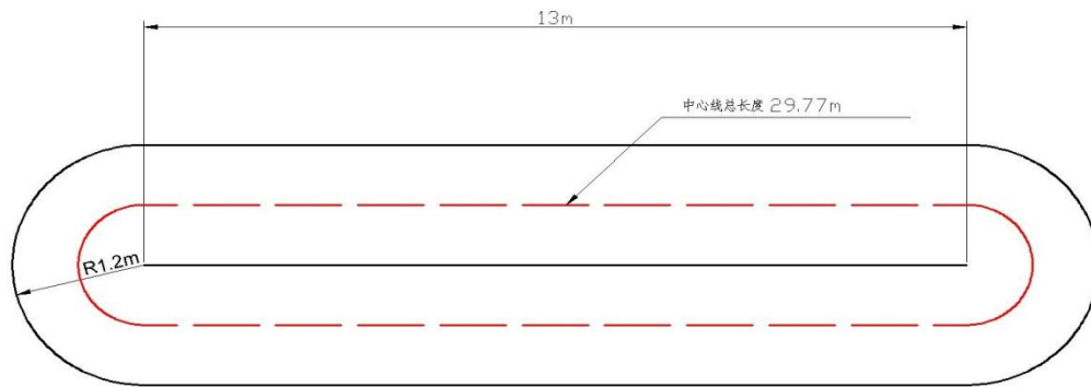
图 5 赛道示意图
